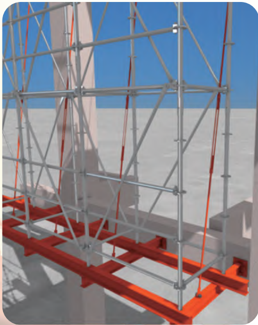
新型装配式外架支撑体系三维图
